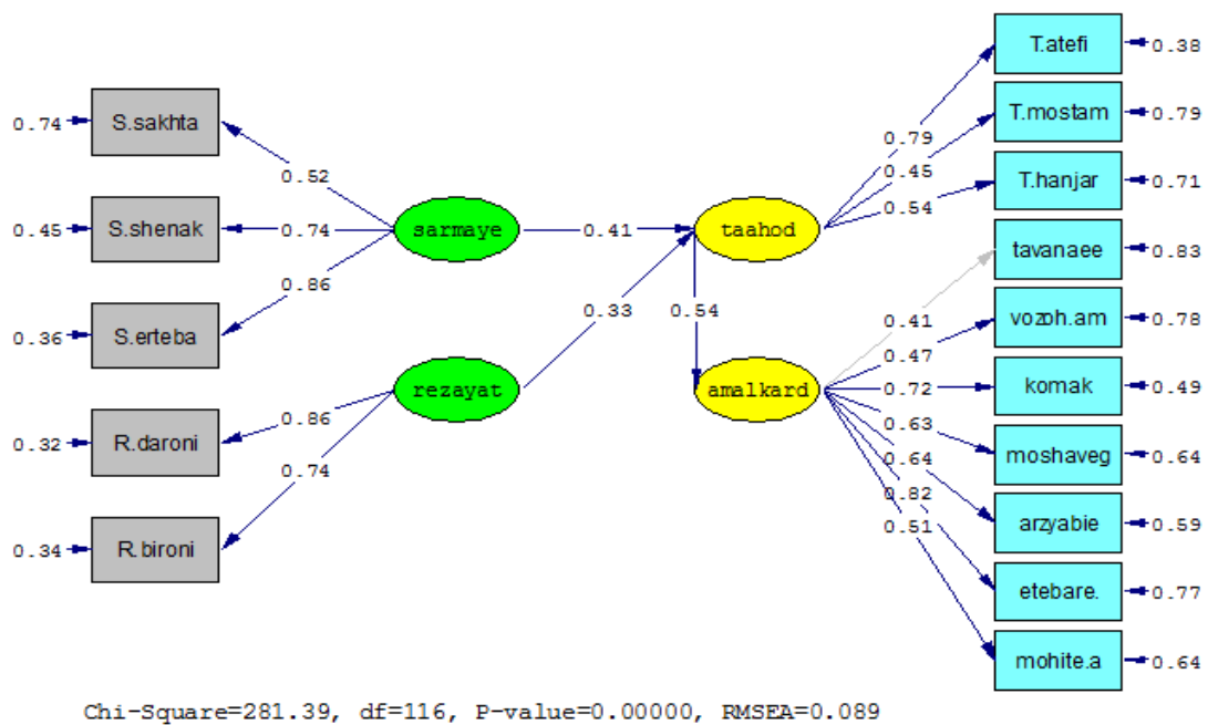
شکل ۲. خروجی لیزرل برای آزمون ضرایب استاندارد شده بتا به همراه سطح معنی‌داری مدل
