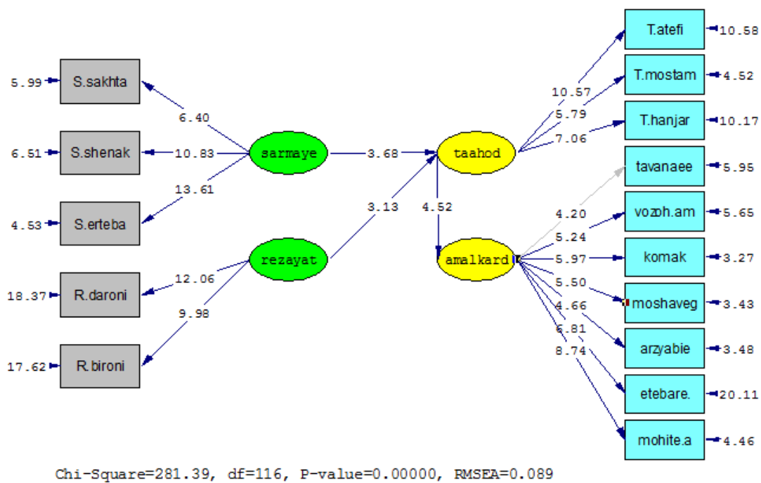
شکل ۳. خروجی لیزرل برای آزمون ضرایب استاندارد T
