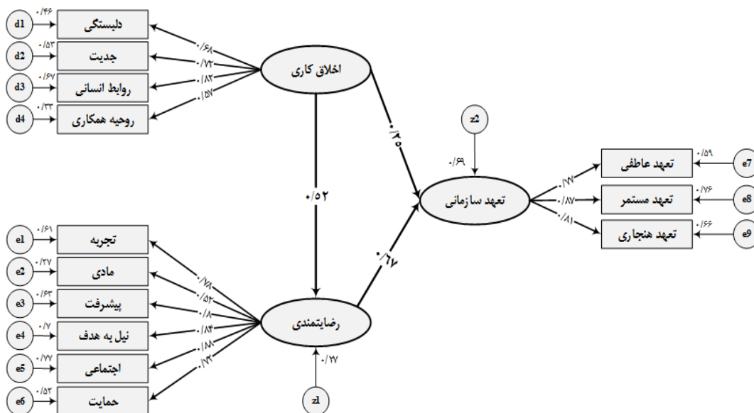
شکل ۲. مدل معادله ساختاری پژوهش به همراه ضرایب تأثیر استاندارد
