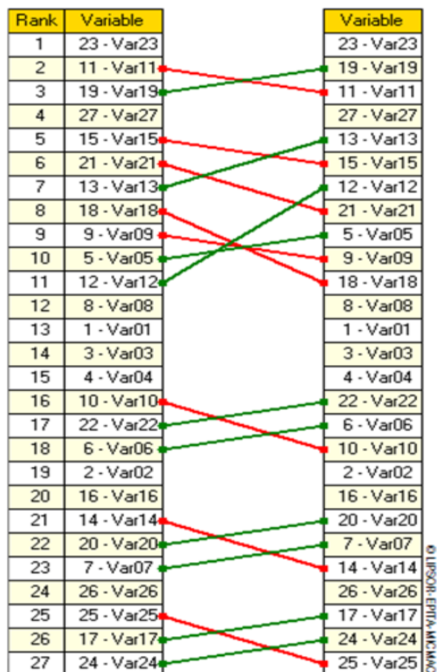
جدول ۵. اولویت بندی پیشران های کلیدی برحسب اثرگذاری مستقیم و غیرمستقیم
