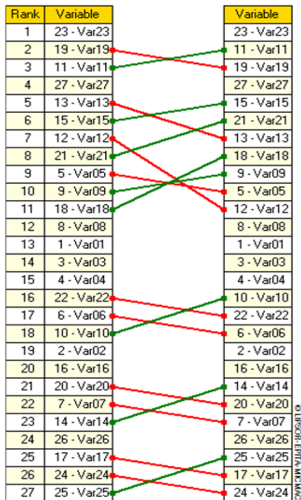
جدول ۶ جدول اولویت‌بندی پیشران‌های کلیدی برحسب اثرپذیری مستقیم و غیرمستقیم
