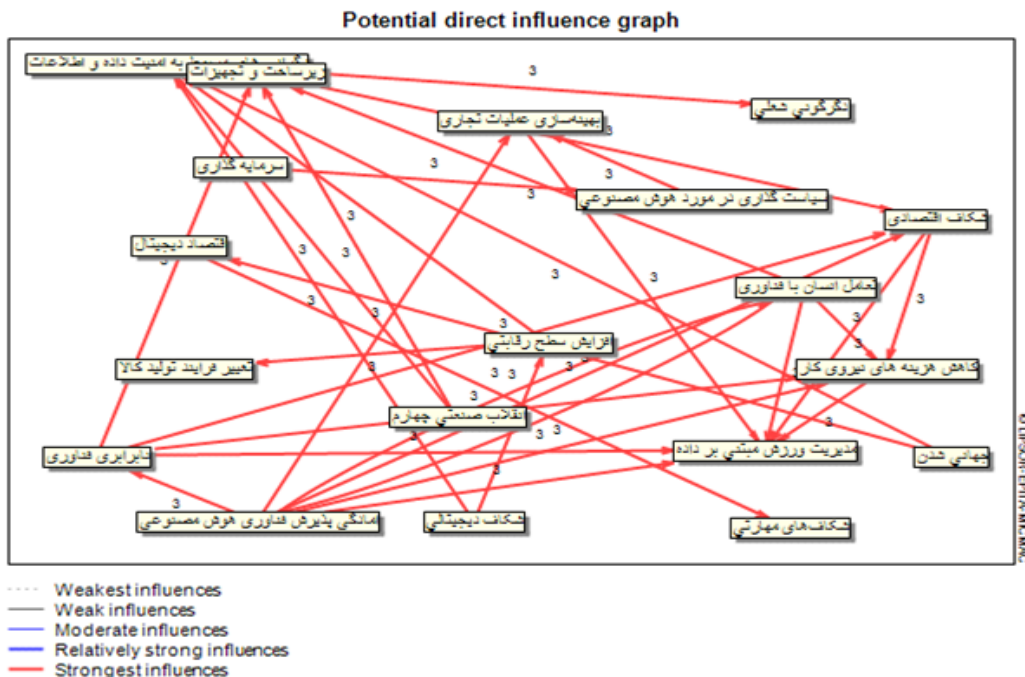
شکل ۴. شدت ارتباط در تأثیرگذاری مستقیم بالقوه پیشران ها (در سطح ۵٪)
