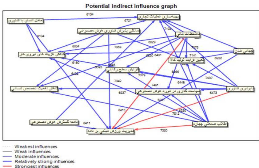
شکل ۵. شدت ارتباط در تأثیرگذاری غیرمستقیم بالقوه پیشران ها (در سطح ۵٪)
